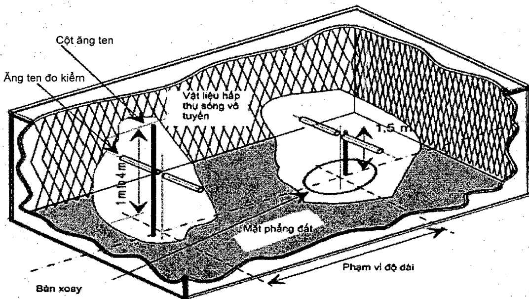
Hình C.2 - Phòng đo kiểm không phản xạ với mặt phẳng dẫn điển hình
