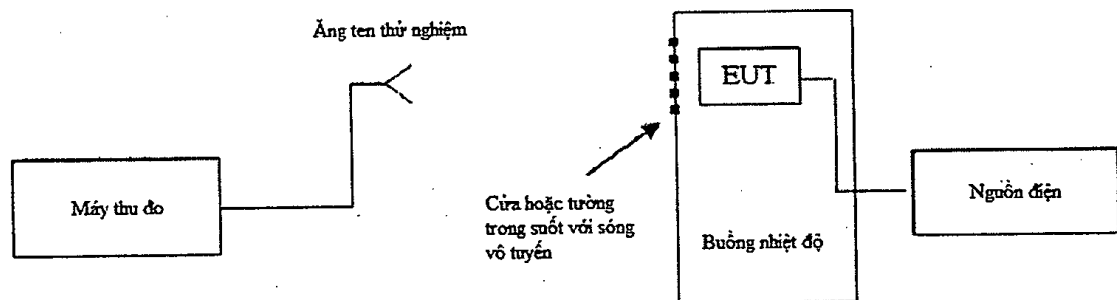
Hình C.3 - Thiết lập điều kiện đo kiểm khác nghiệt
