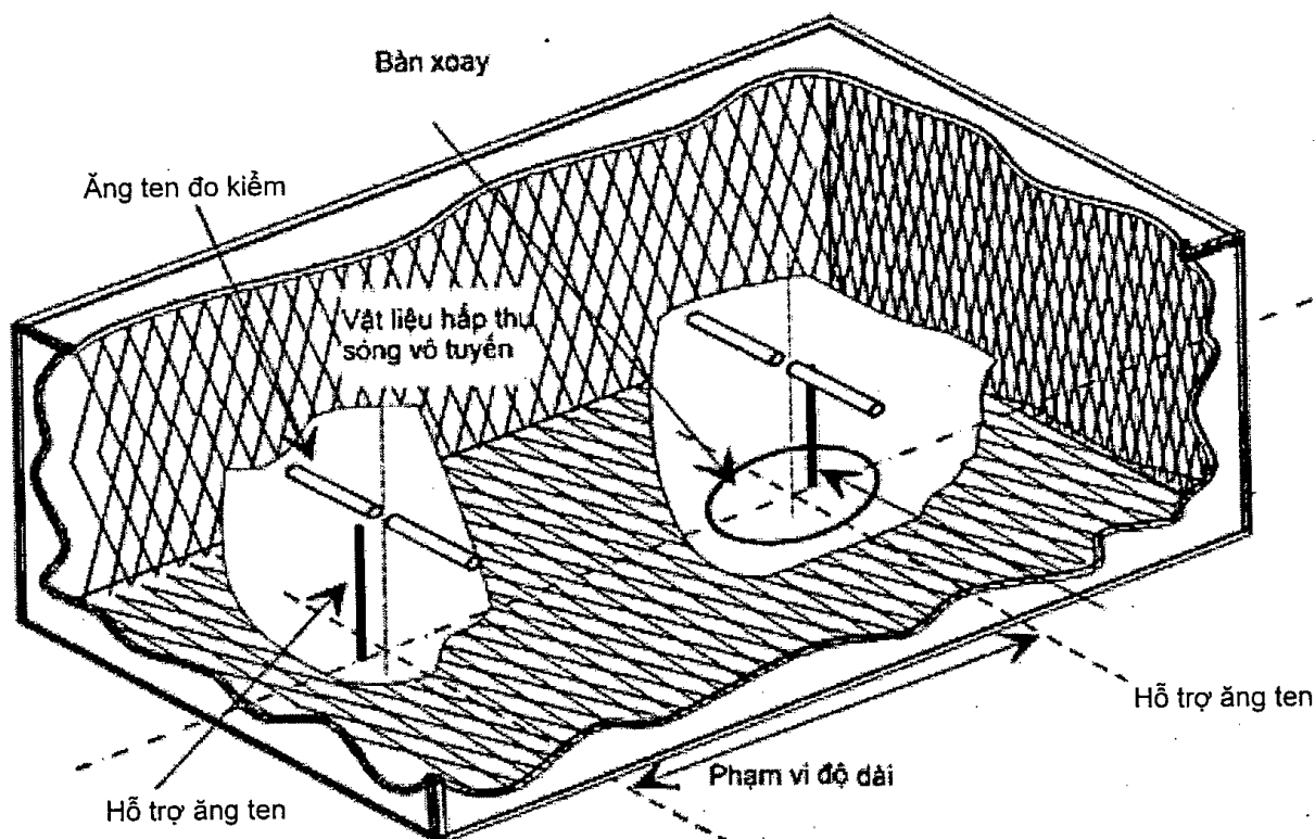
Hình C.1 - Phòng đo kiểm không phản xạ điển hình
